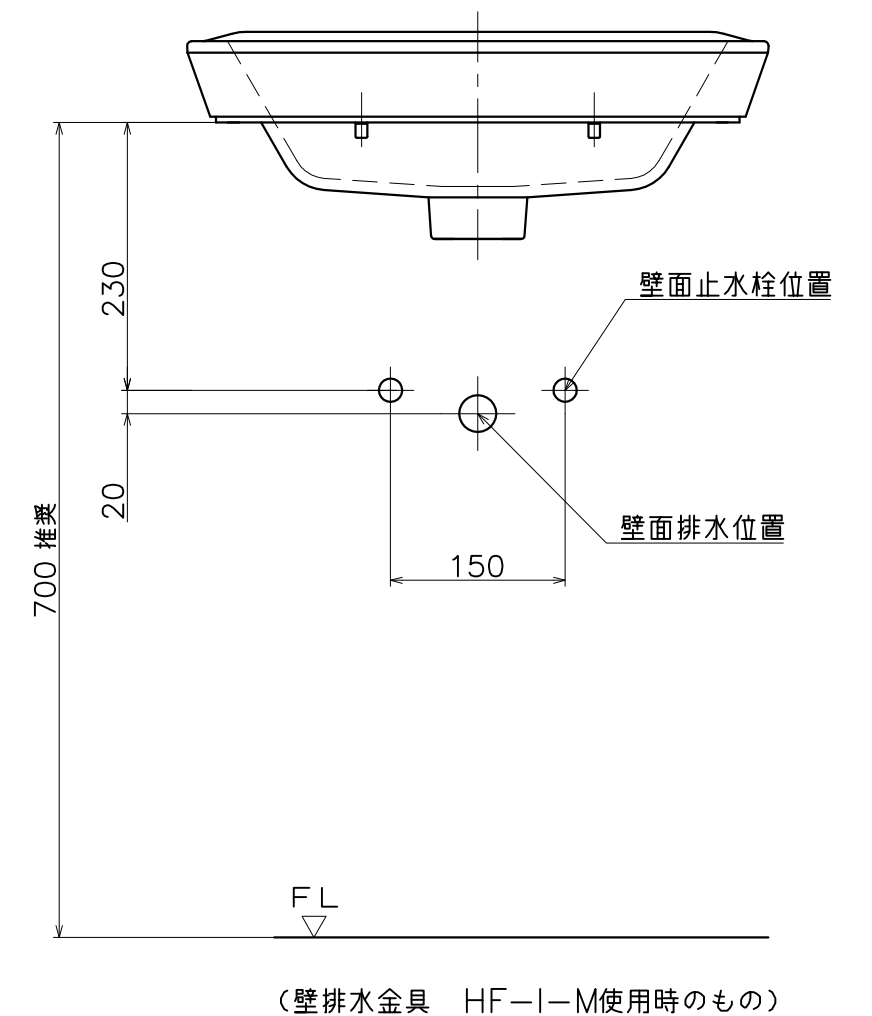
取付参考図
