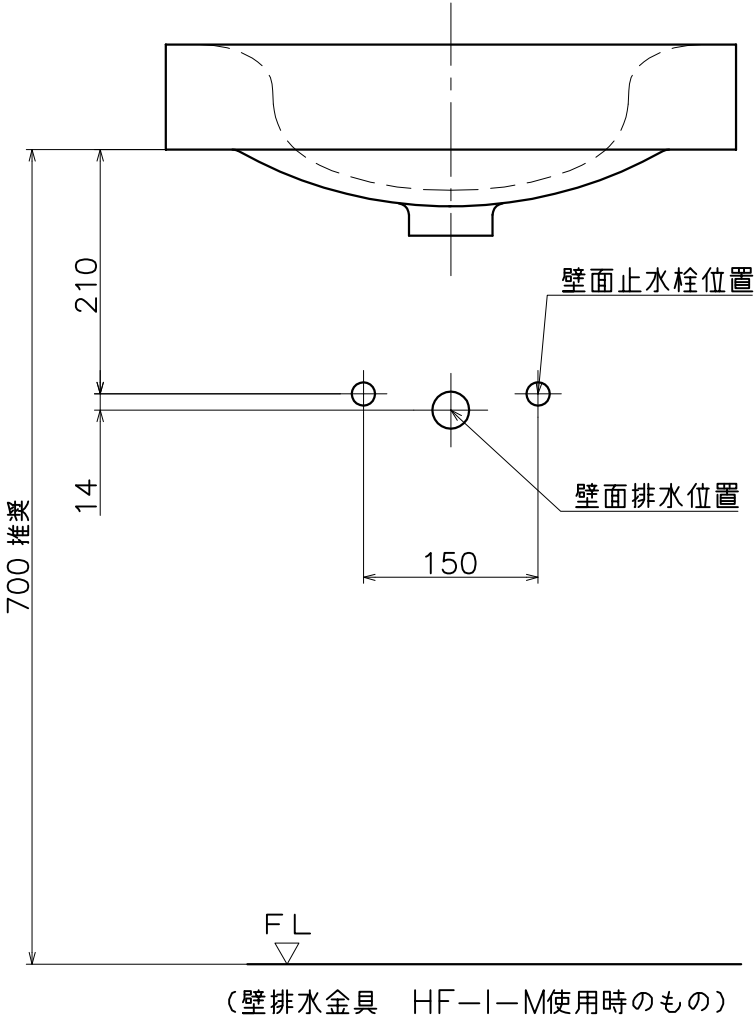
取付参考図
