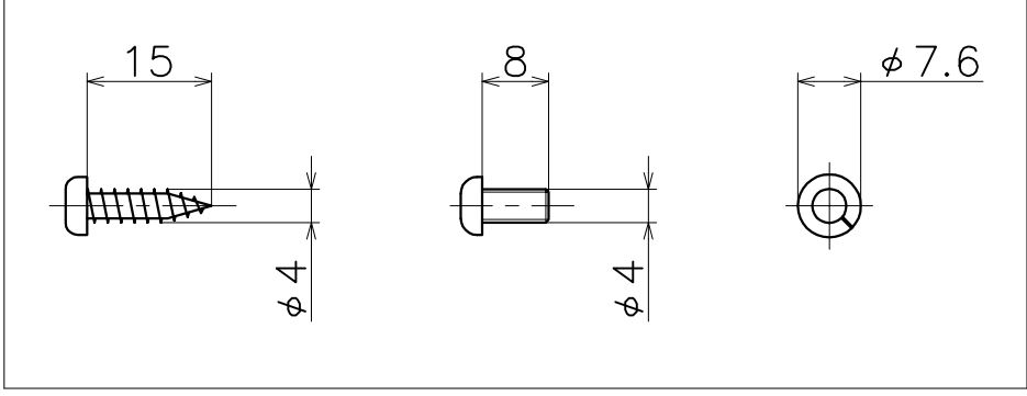
付属ねじ
