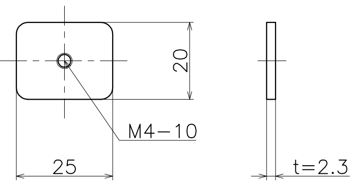
角ナット
