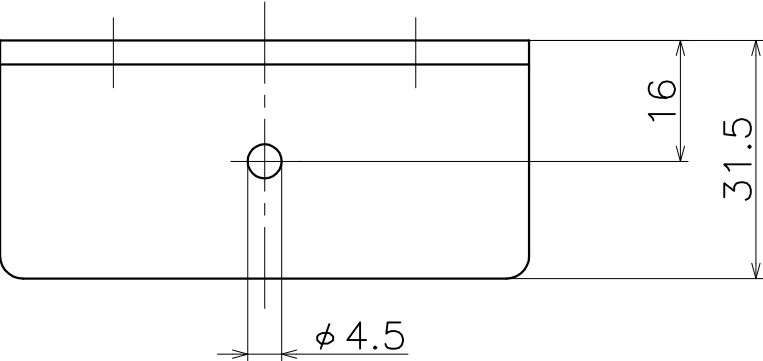
コネクター
