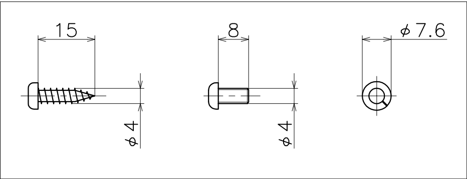
付属ねじ
