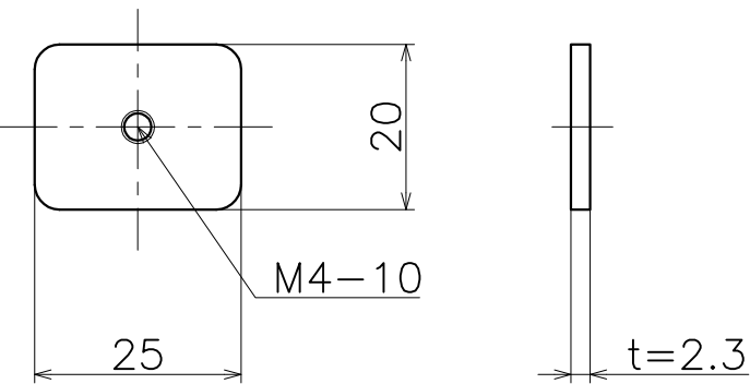
角ナット
