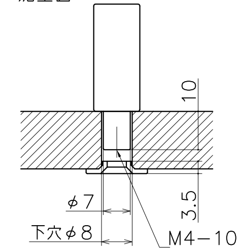
施工図
