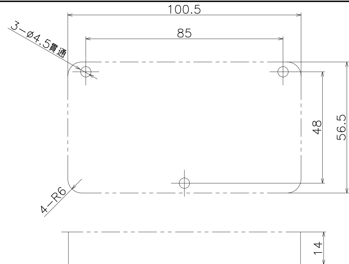
切欠図 (S=1:1)
