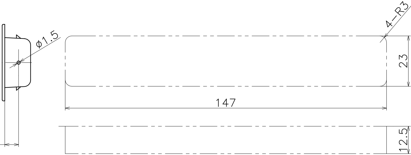
切欠図（S=1:1）
