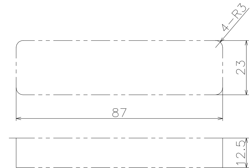
切欠図 (S=1:1)
