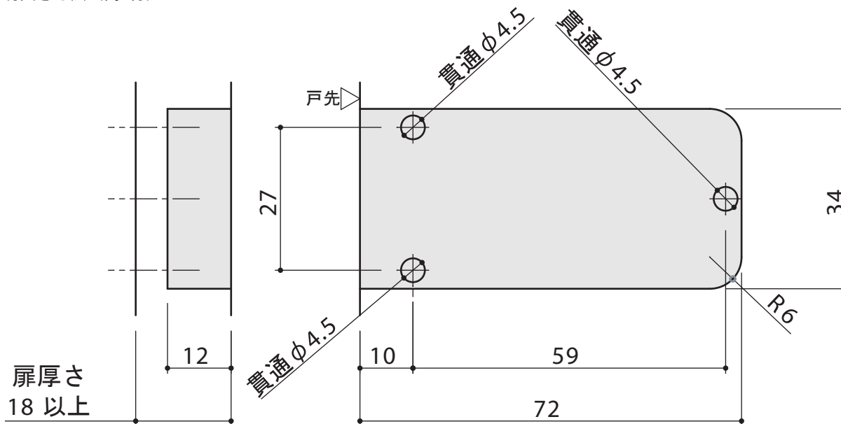
PC-397切欠き寸法（角R付）
